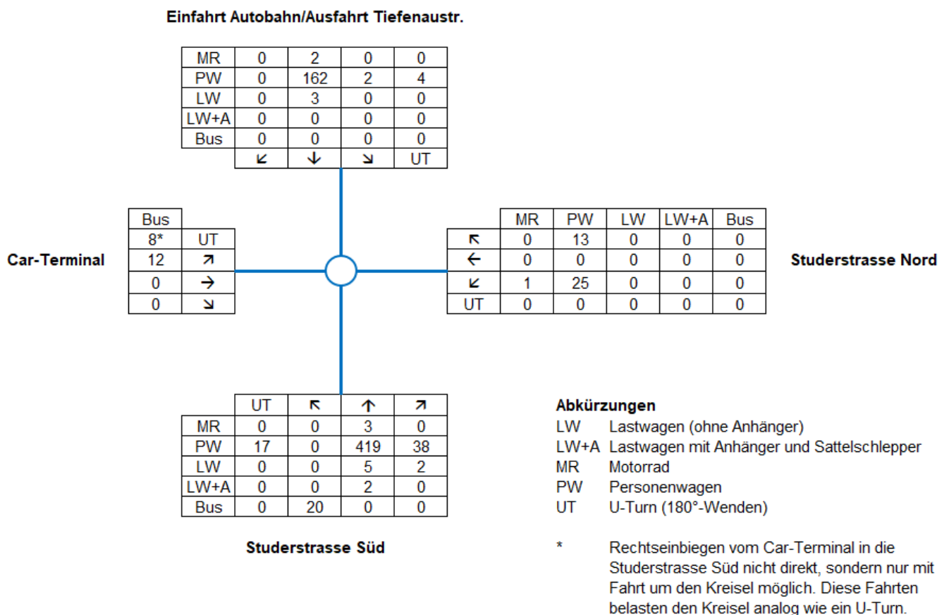
Abbildung 3: Verkehrsmengengerüst Abendspitzenstunde
