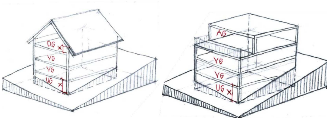
Dach-, Voll- und Untergeschoss
