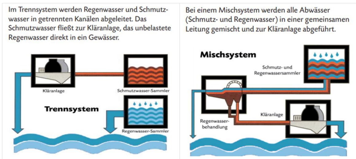
Abbildung 1: Darstellung Entwässerungssysteme
