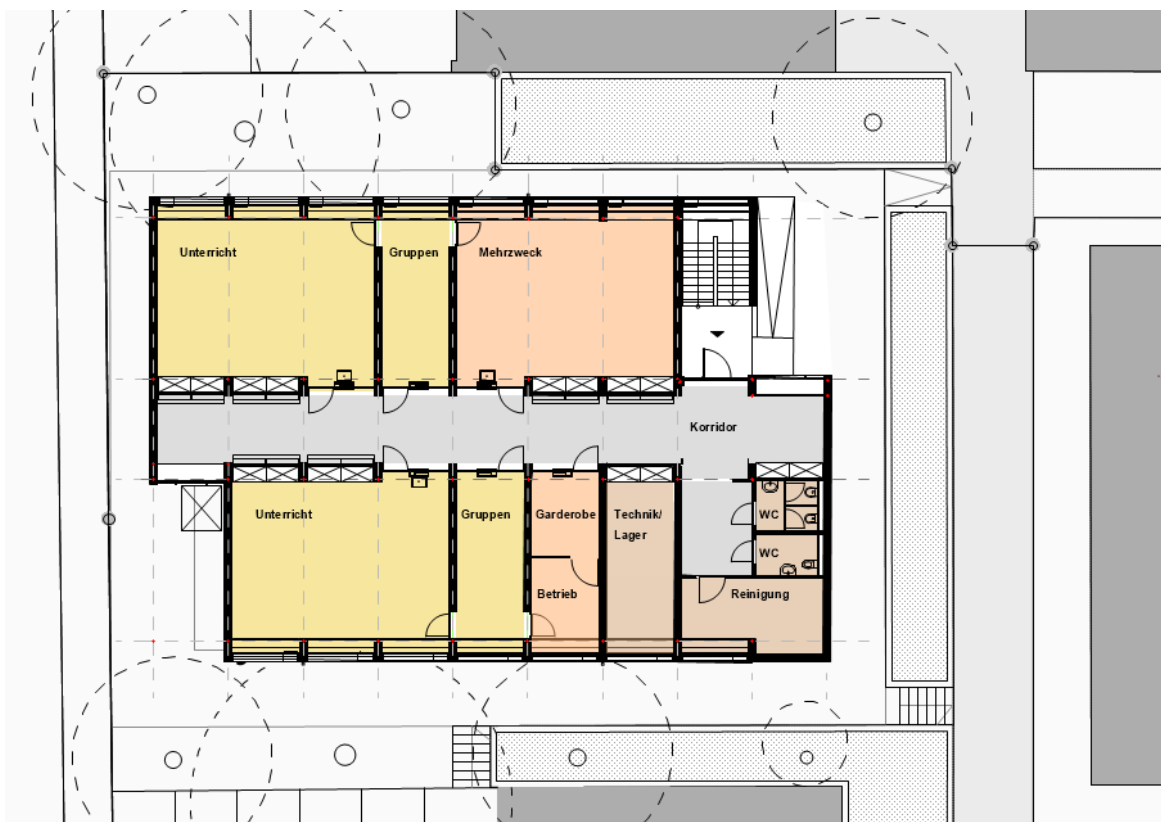
Abb.7: Grundriss Provisorium Steigerhubel (Stand Machbarkeitsstudie)
