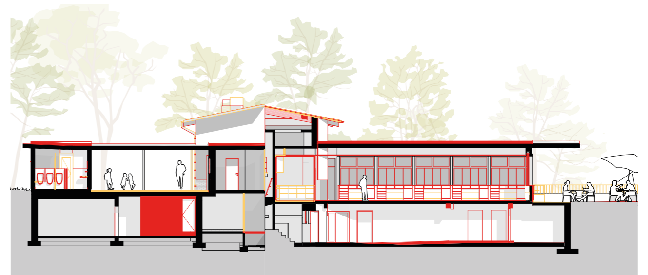
Längsschnitt
