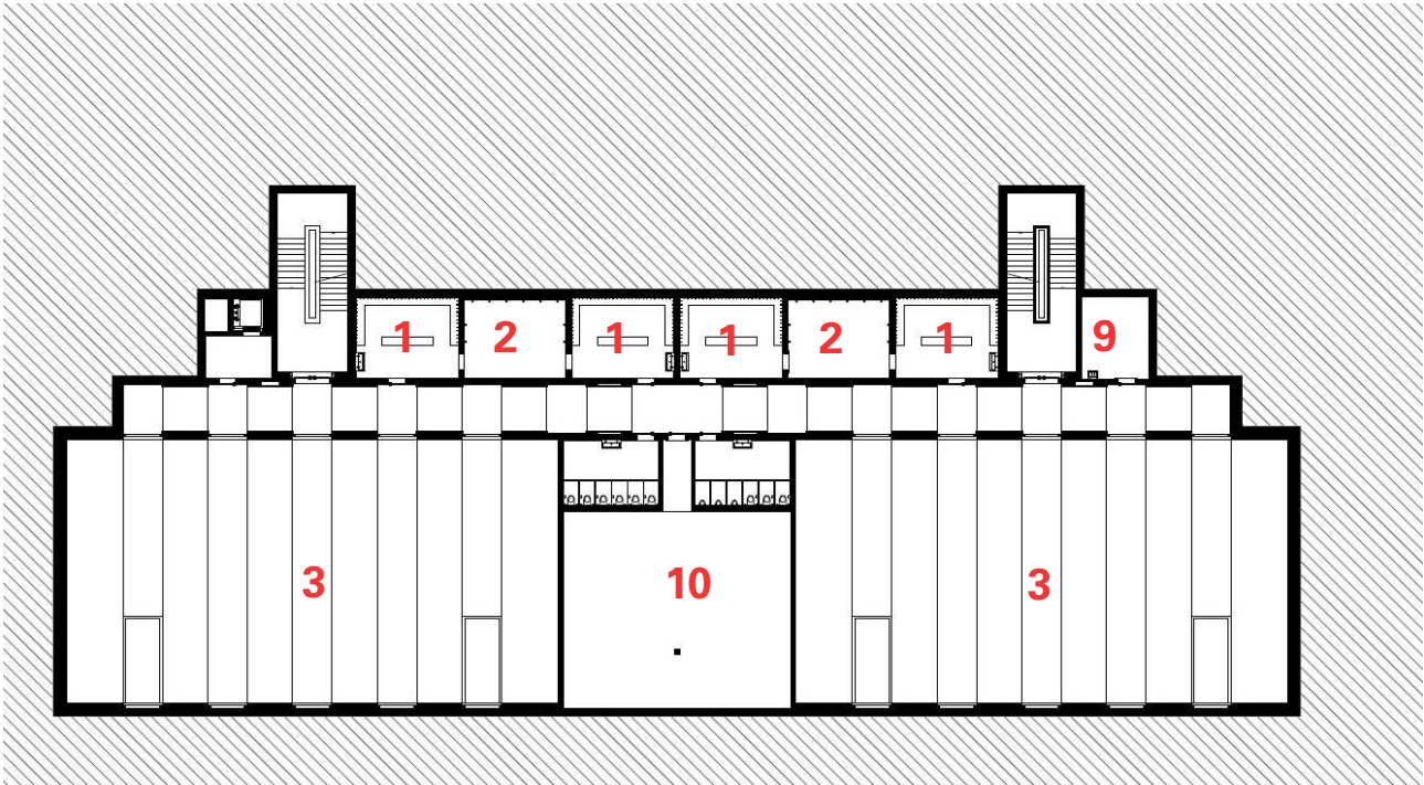
2. Untergeschoss
