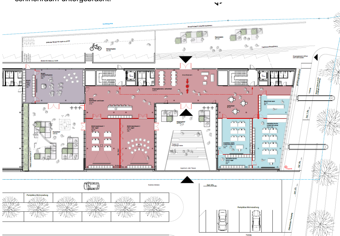
Situationsplan mit Hofgeschoss
