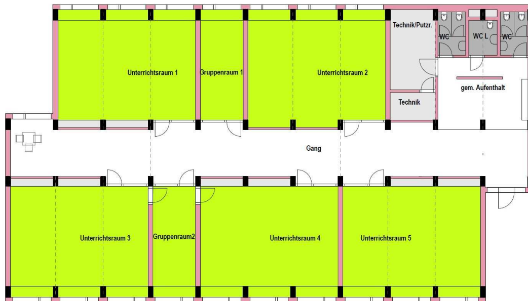
Grundrissbeispiel Projekt Brünnpavillons
