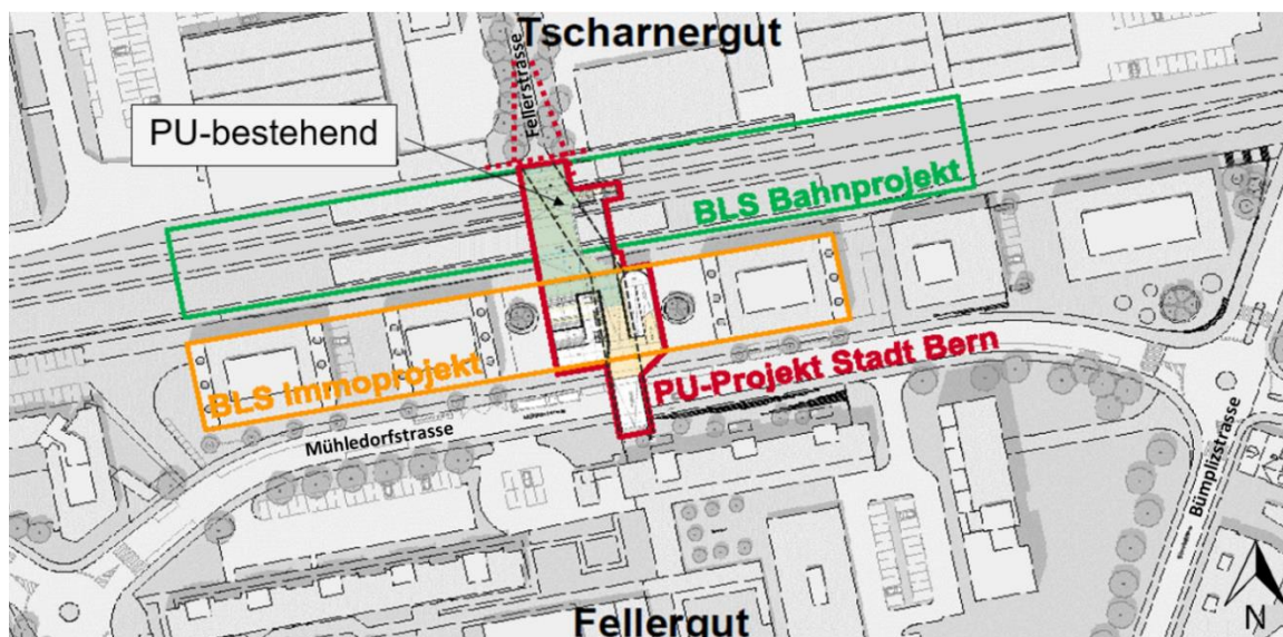
Abbildung 1 Übersicht Projektteile beim S-Bahnhof Bern Bümpliz Nord (Stand Vorprojekt)
