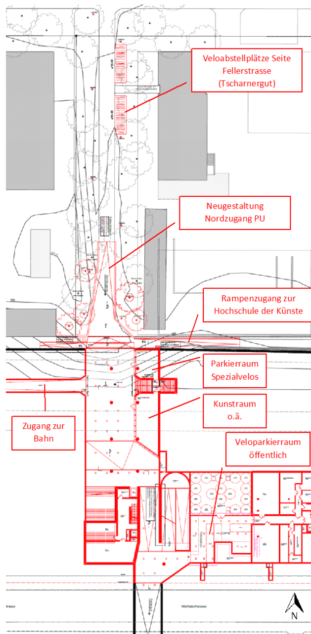
Abbildung 4: Ausschnitt aus Übersichtsplan des geplanten Projekts Verbreiterung und Aufwertung Personenunterführung Bümpliz Nord (Abbildung aus dem Vorprojekt; Stand 21. Dezember 2021)
